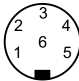
6 pins DIN 45322
