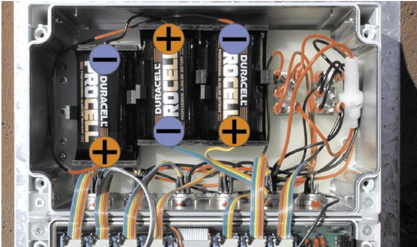
Interne Batterien
